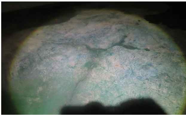
지하2층 하부슬래브 물탈들뜸
