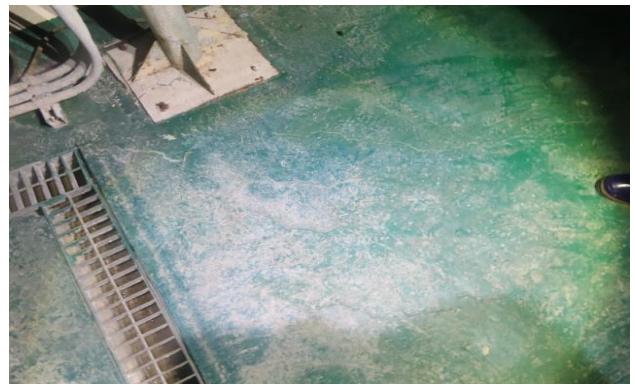
지하2층 하부슬래브 망상균열
