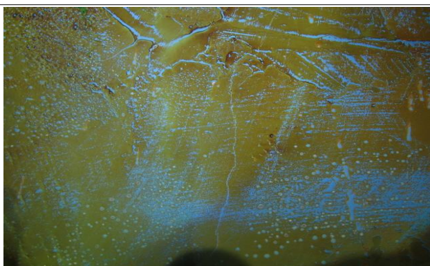
배수지 2지 벽체 균열(0.3mm미만)
